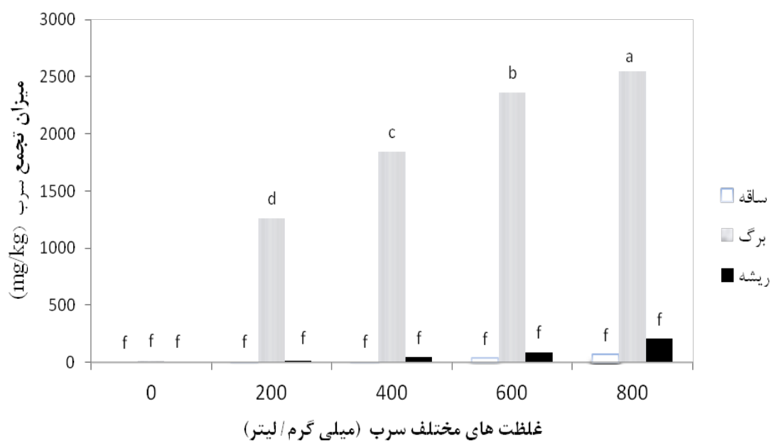
شکل ۱- میانگین اثر متقابل غلظت سرب بر میزان تجمع سرب در اندامها (حروف غیرمشترک اختلاف معنی دار را نشان می دهد p < 0.05 ): ارزیابی توانایی گیاه پالایی گونه عسلی ( Alyssum maritimum ) در پالایش خاکهای آلوده به سرب
