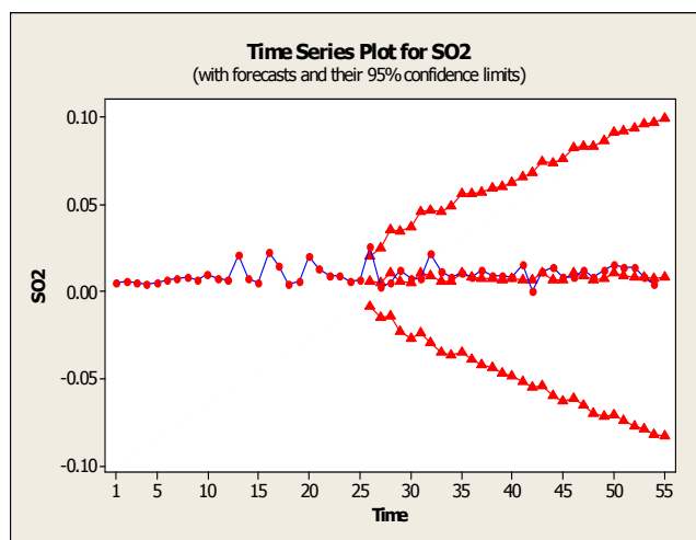
(g) SO2
