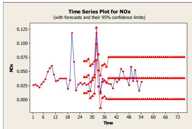
(e) NOx
