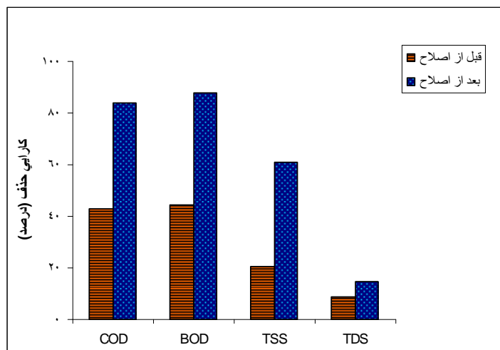
نمودار ۱ - مقایسه‌ی بازده حذف COD, BOD 5 , TSS و TDS در سامانه‌ی بی‌هوای
