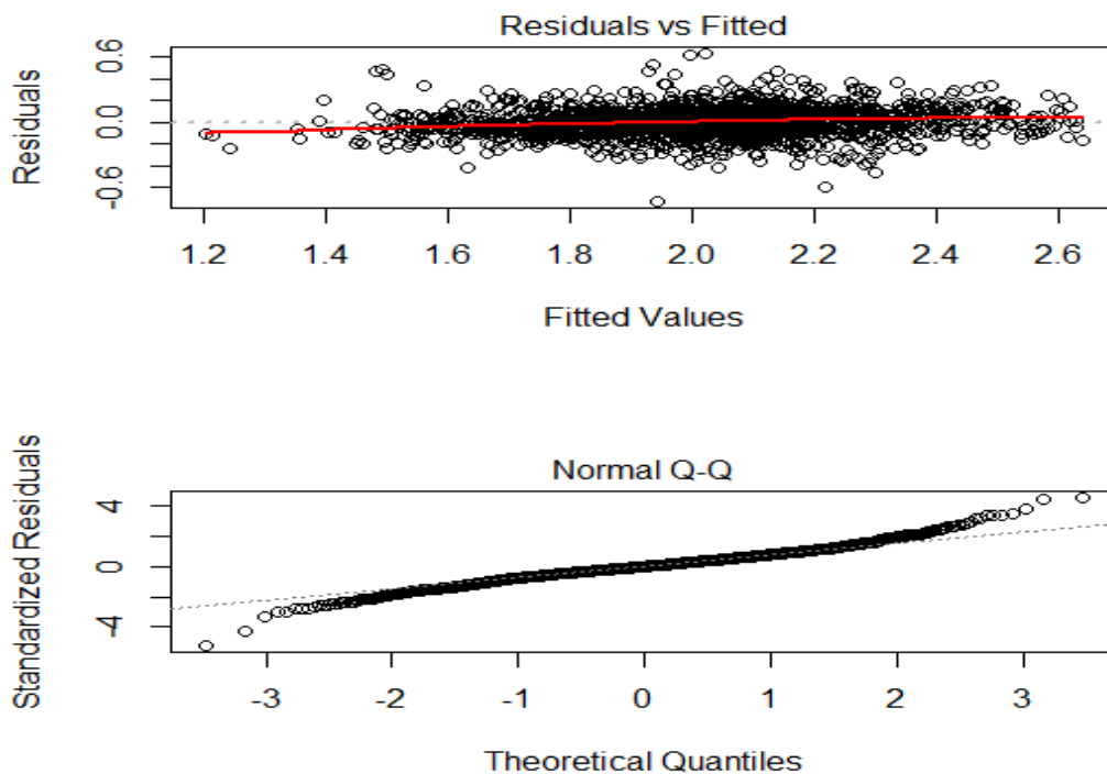
شکل ۱- نمودارهای بررسی مناسبیت مدل توأم
