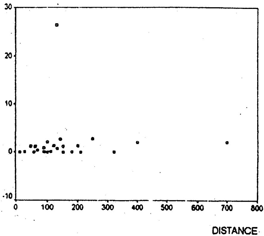
نمودار ۴- مقادير اندازه گيري شده نيتريت در چاههای مورد بررسی در منطقه غرب تهران و مقایسه آنها با فواصل محل تخلیه فاضلاب
