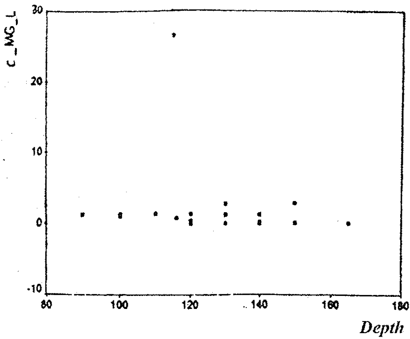
نمودار ۳- تغییرات غلظت نیتريت در چاههای با عمقهای مختلف در منطقه غرب تهران در سال ۱۳۷۷
