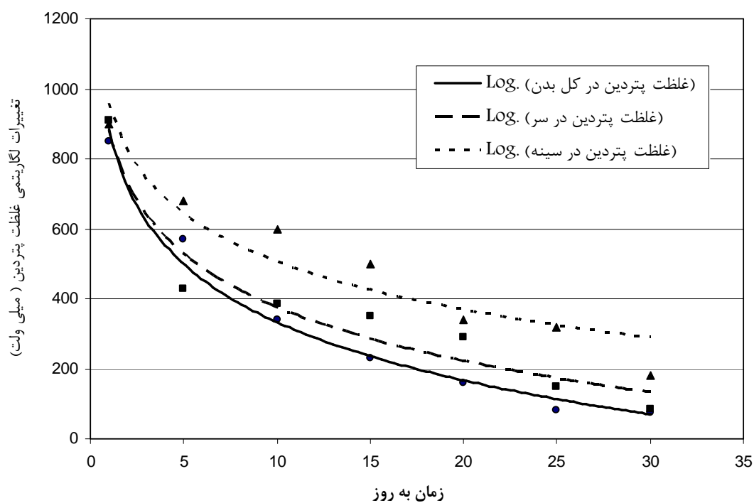
نمودار ۲- مقایسه تغییرات غلظت پتریدین استخراج شده از کل بدن، سر و سینه پشه های ماده آنوفل استغفسی طی ۳۰ روز با پر بود زمانی ۵ روزه، سر و یا سینه پشه ها در گروه های ۱۰ تایی بصورت جداگانه در ۱۰۰ میلی لیتر بافر و کل بدن هر ده عدد آنوفل ماده نیز در ۶۰۰ میلی لیتر بافر هموژنیزه کننده قرار داده شد و پس از هموژنیزه، سانتریفیوژ و فیلتر شدن، ۱۰ میکرو لیتر از هر محلول به سیستم HPLC تزریق شد.
