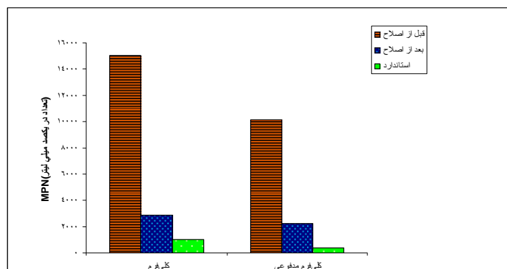
نمودار ۶- مقایسه‌ی خروجی نهایی کلیرم کلیفرم‌ها و کلی‌فرم‌های مدفوعی تصفیه‌خانه با استانداردهای ملی بر حسب تعداد کلی‌فرم در یکصد میلی‌لیتر (قبل و بعد از اعمال تغییرات)
