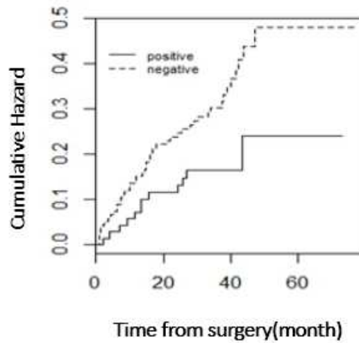
شکل ۲- تابع مخاطره بروز متاستاز بیماران سرطان پستان، به تفکیک عوامل پیش‌آگهی دهنده: مراجعه کنندگان به بیمارستان فیاض بخش تهران، ۸۶-۱۳۸۴
