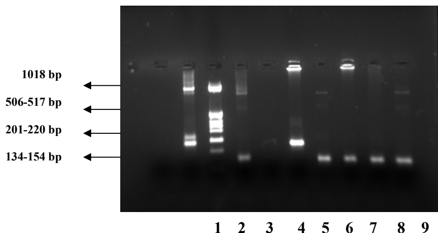
تصویر ۱: بررسی از نظر آلودگی به اسپیروزوئیت انگل مالاریا در پشه های آنوفل استفنی و آنوفل کولیسفاسیس باندهای 205 bp و 120 bp بترتیب نشانگر آلودگی پشه به P. falciparum و P. vivax می باشد. ردیف ۱، کنترل P. falciparum ؛ ردیف ۲، مارکر 1 kbp ladder؛ ردیف ۳، کنترل P. vivax ؛ ردیف ۴، کنترل منفی؛ ردیف ۵، P. falciparum ؛ ردیف ۶-۹، P. vivax ؛
